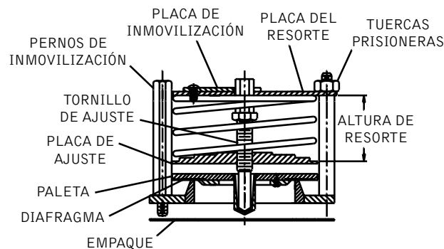
DETALLE DEL PAQUETE DE RESORTE
