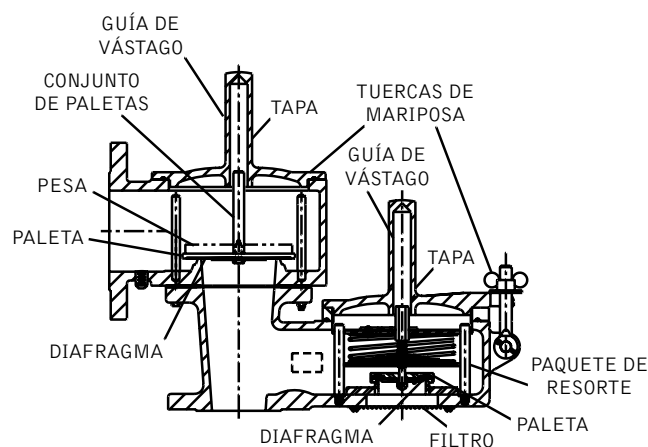
VACÍO CON CARGA DE RESORTES/PRESIÓN CON CARGA DE PESAS
